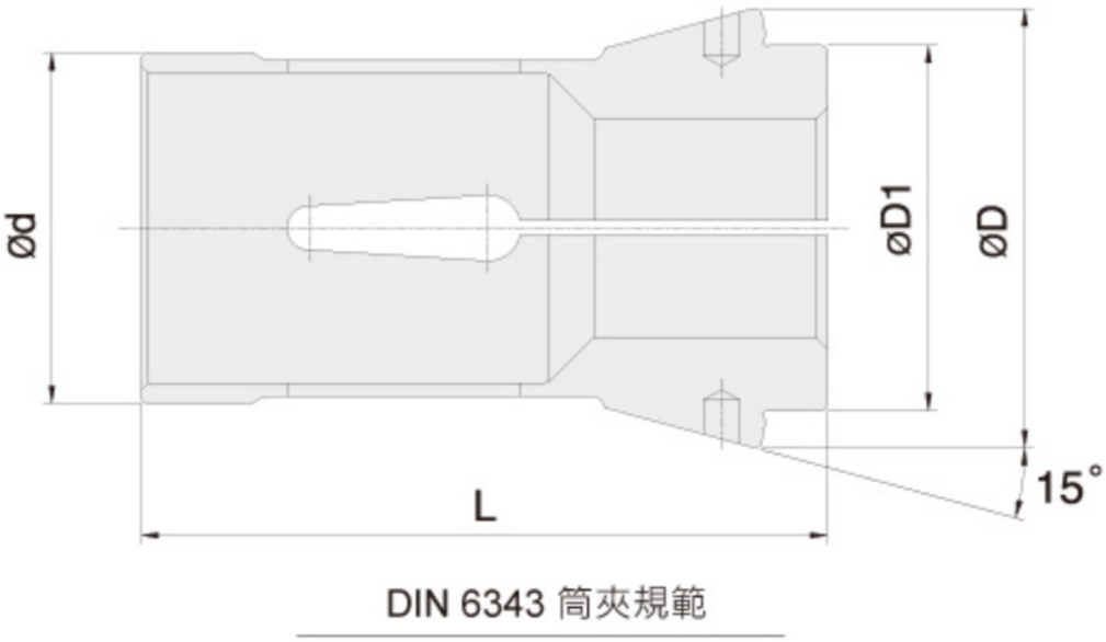
DIN 6343 筒夾規範
